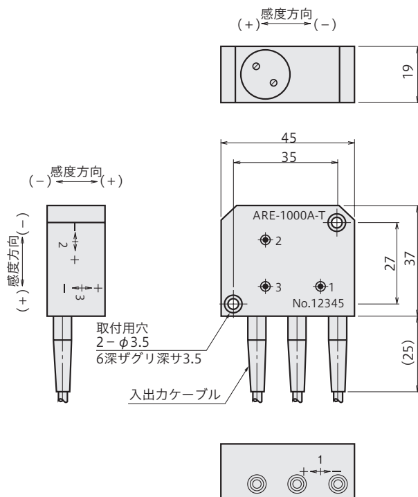
外観寸法図
