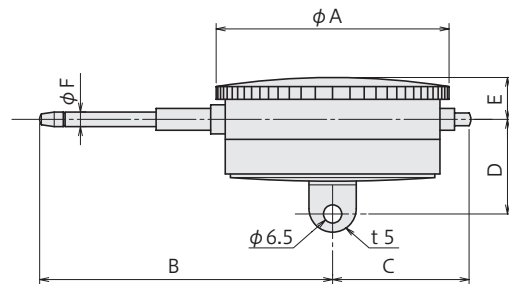
DDP-10~30A
