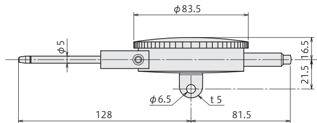
DDP-50A
