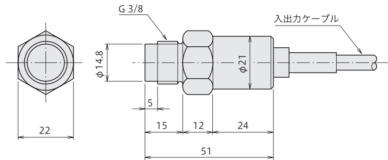
外観寸法図
